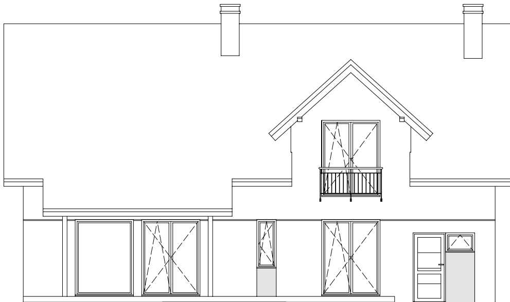
ELEWACJA OGRODOWA
